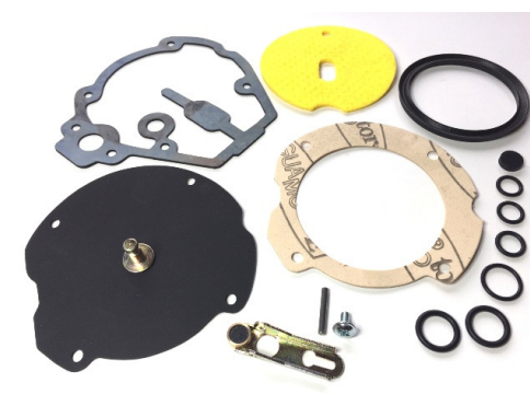
4263 LANDI LI 02
